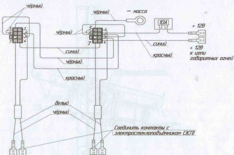
Рис. 3. Схема подключения электростеклоподъемников к бортовой сети автомобиля.
