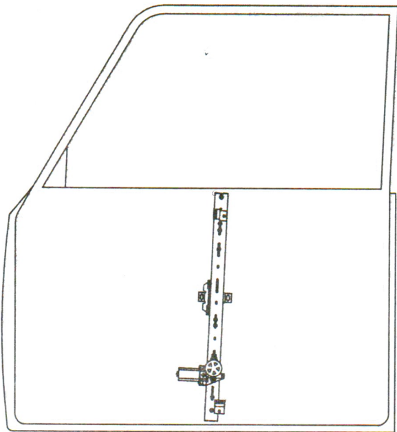
рис. 1. Ориентация стеклоподъемника
